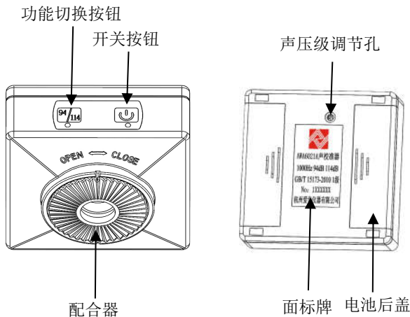
图 1 校准器结构示意图
