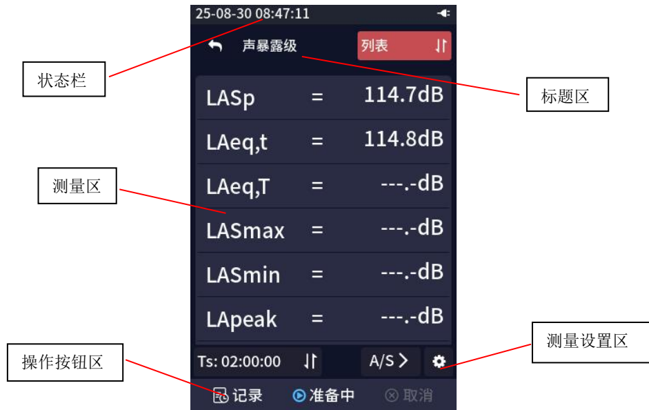
图 6-3-8-1 声暴露级列表界面
