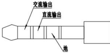
图 4-1-5 立体声插头引脚
