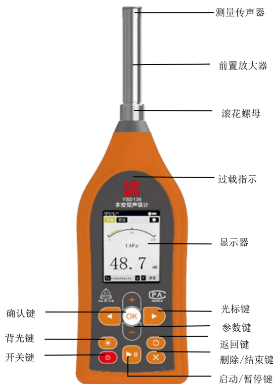
图 4-1-1 仪器正面
