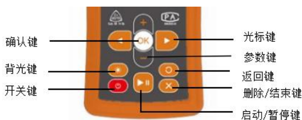
图 4-2-1 按键功能
