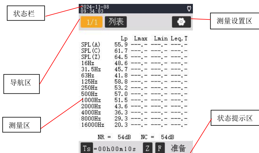
图 6-2-5-1 1/1 OCT 列表
