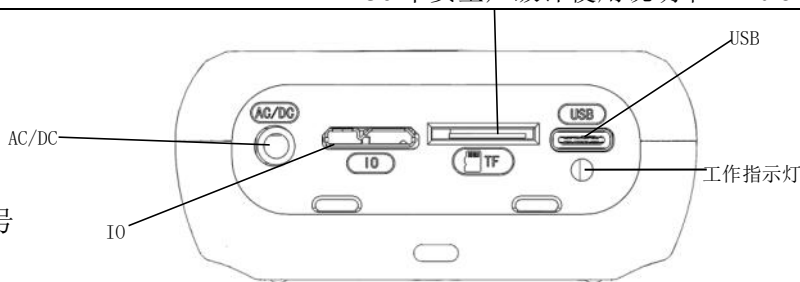
图 4-1-4 底部接口
