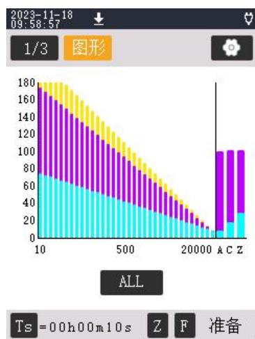
图 6-2-6-2 1/3 OCT 图形
