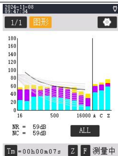
图 6-2-5-2 1/1 OCT 图形
