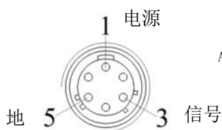
图 4-1-3 X9 插座
